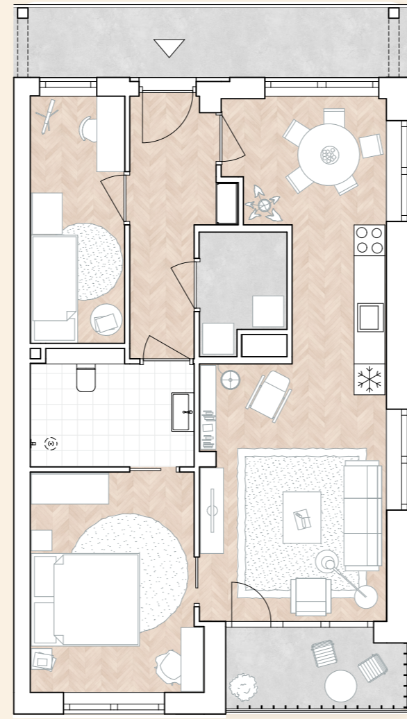
Royale rolstoelgeschikte woning
